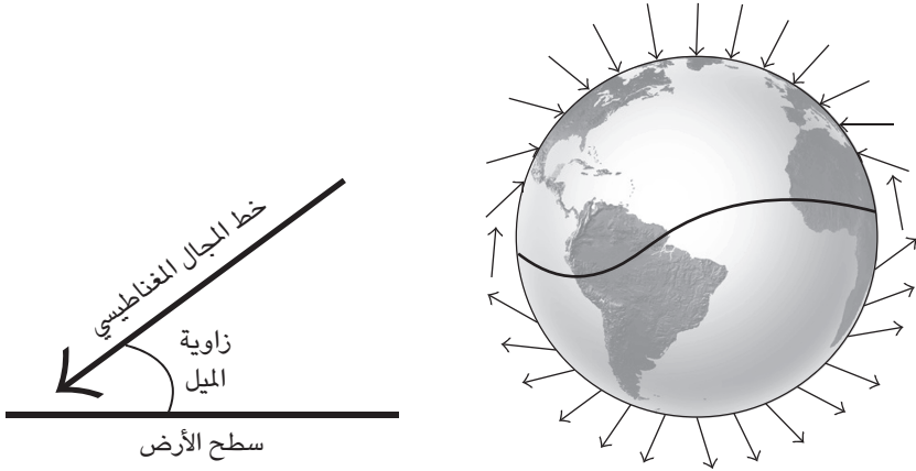
شكل ٦-١: خطوط المجال المغناطيسي للأرض وزاوية الميل.
